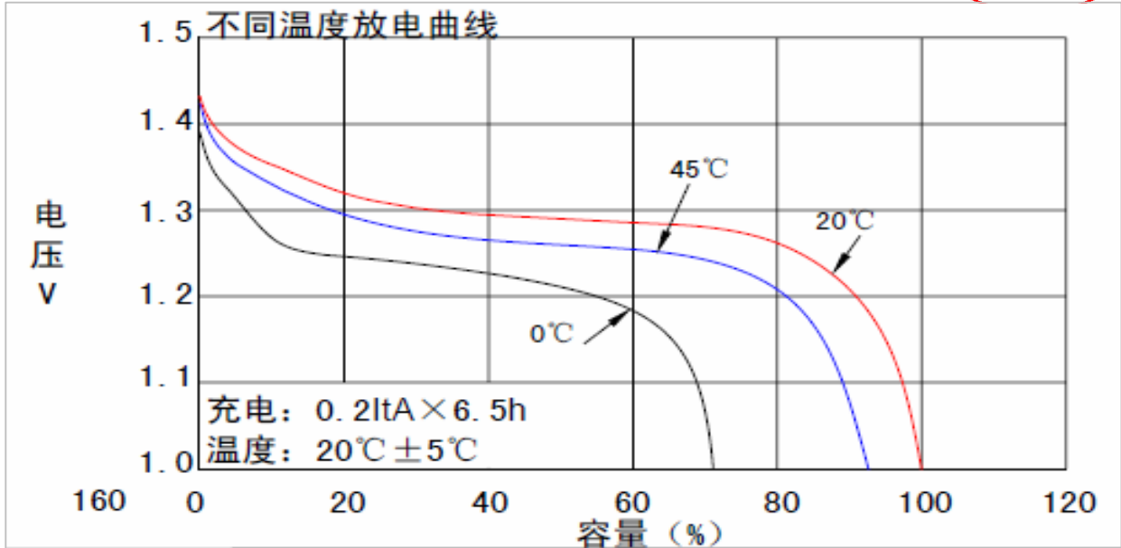
特征曲线
