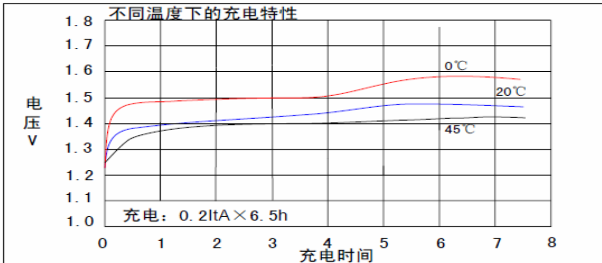
特征曲线
